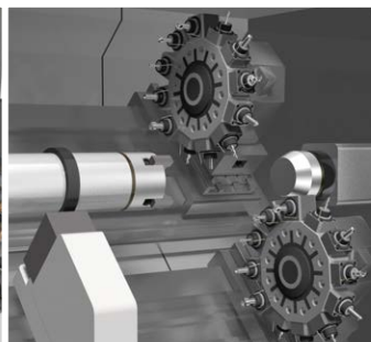
旋盤複合機 Multi-tasking lathe
